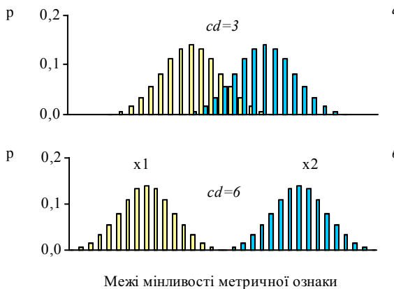
Рис. 2. Характер мінливості деякої метричної ознаки за двох рівнів відмінностей між вибірками: CD=3 (а) та CD=6 (б). При CD=3 третина діапазону мінливості недиагностична (а), при CD=6 гіатус повний (б). У першому випадку x_1 = \min_2 , \max_1 = x_2 ; у другому – збігаються лише крайні значення ознак: \max_1 = \min_2 .
