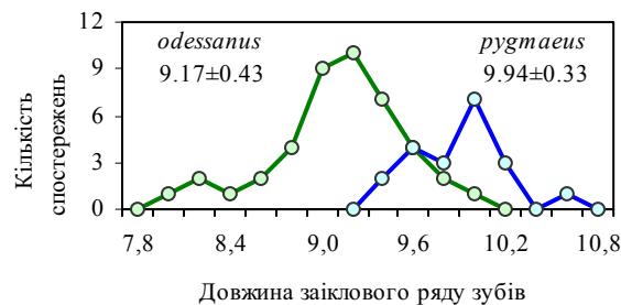
Рис. 1. Розподіл значень метричної ознаки у двох близьких видів: аналіз мінливості довжини зубного ряду (верхні заїклові зуби, P^4M^3 ) у дорослих особин двох видів ховрахів з території України за зразками з колекції ННПМ: ховрах подільський ( Spermophilus odessanus ) і ховрах малий ( S. pygmaeus ). Коефіцієнт дивергенції у цьому випадку CD=1,89 .
