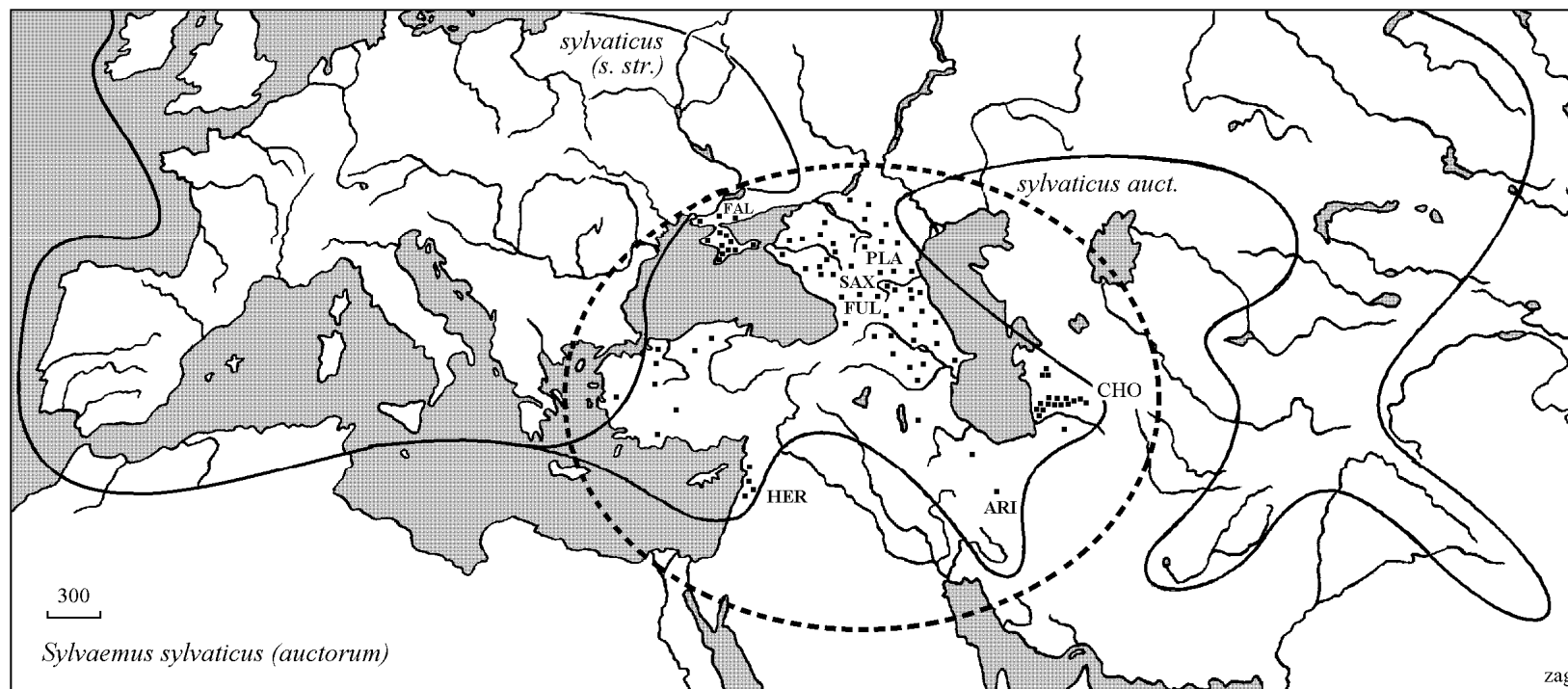
Рис. 1. Ареал надвида “ Apodemus sylvaticus ” в области Древнего Средиземья и распространение степных форм группы Sylvaemus falzfeini (южная Украина) — fulvipectus (Кавказ) — chorassanicus (Копетдаг) — arianus (Персия) — hermonensis (Малая Азия). Контурсы ареала прежнего политипического вида S. sylvaticus приводятся по карте из сводки Дж. Корбета (Corbet, 1978), восточная граница ареала S. sylvaticus s. str. — по И. Загороднюку (1993). Буквами обозначены типовые местонахождения таксонов, относимых здесь к виду Sylvaemus arianus .
