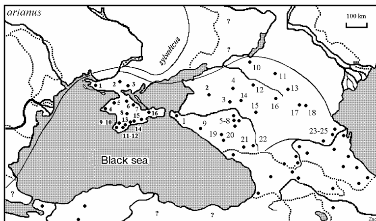
Рис. 4. Детали географического распространения степной мыши ( Sylvaemus arianus ) на территории Восточной Европы и прилегающих районов Кавказа и южного Причерноморья. Сплошной линией обозначена юго-восточная граница ареала S. sylvaticus . Цифрами отмечены известные места регистрации степной мыши в Украине (№ 1–16, S. a. falzfeini ) и северо-кавказском регионе (№ 1–25, S. a. fulvipectus ; см. текст). Ненумерованные пункты находок в южном Дагестане, Грузии, Азербайджане и Армении — по П. Свириденко (1936) и Н. Воронцову с соавт. (1992), находки S. a. hermonensis в Анатолии — по данным М. Филиппуччи с соавт. (Filippucci et al., 1996).
