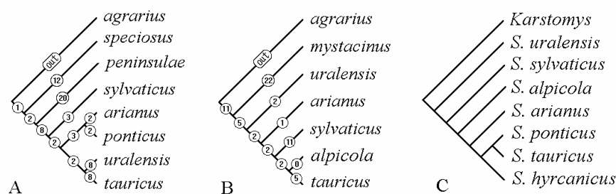
Рис. 3. Кладистические отношения западно-палеарктических Apodemus auct. на основании данных по аллозимной изменчивости мышей, представленных в статьях С. Межжерина и А. Зыкова (1991, А: 148 аллелей 36 локусов), М.-Г. Filippucci (1992; В: 119 аллелей 33 локусов) и вероятная схема таксономических отношений Sylvaemus (С). Индийские rusiges и wardi не рассматриваются. Цифрами отмечено число апоморфий (только аллели, характерные для каждой клады в целом).
