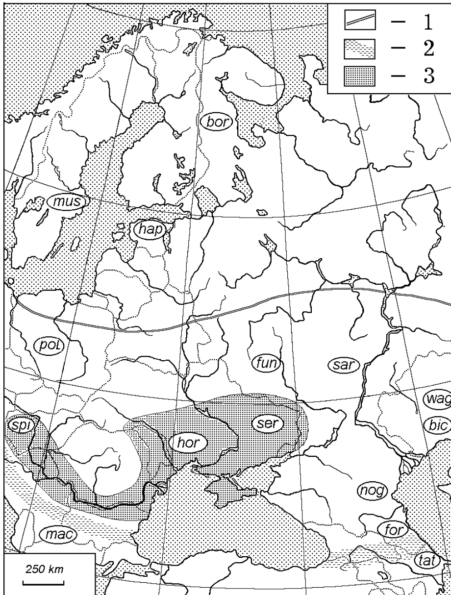
Рис. 1. Типовые местонахождения восточноевропейских форм группы Mus musculus (s. l.), северная граница сезонных экзоантропных популяций Mus musculus (1), зона интерградации musculus—domesticus (2) и область распространения курганчиковых мышей (3). Типовые местонахождения обозначены тремя первыми буквами латинских названий таксонов.
