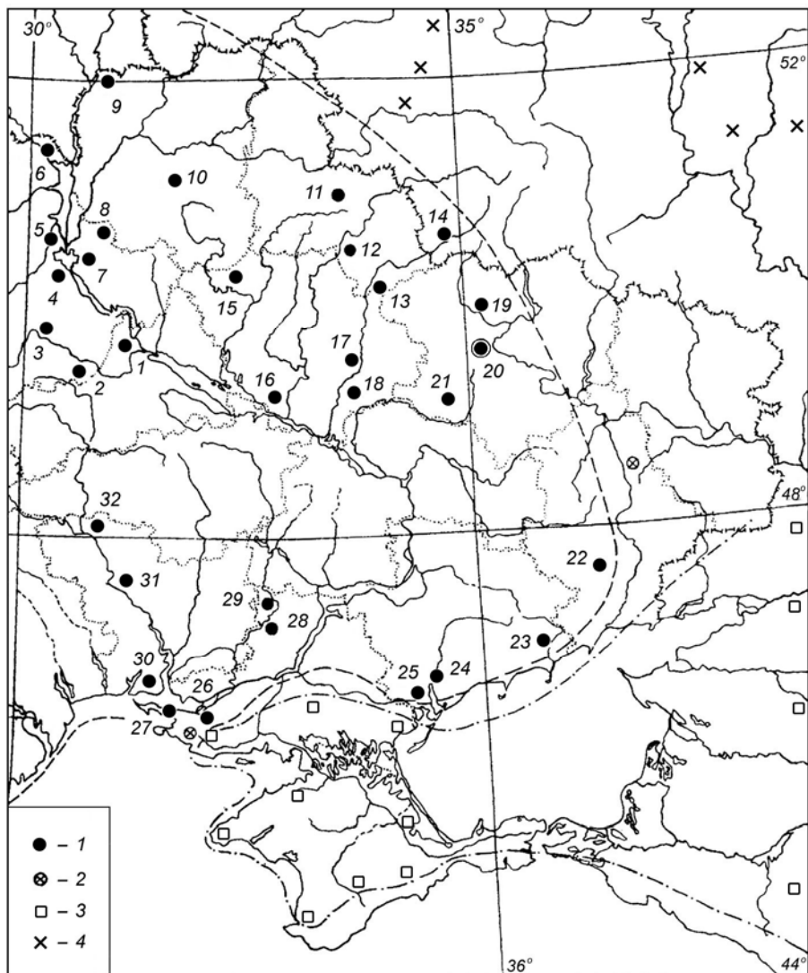
Рис. 3. Места находок и предполагаемые пределы географического распространения Sylvaemus sylvaticus в Восточной Европе к востоку от 30-го меридиана. Номера пунктов соответствуют приводимым в тексте: N 20 — типовое местонахождение S. s. charkovensis . Обозначения: 1 — проверенные находки S. sylvaticus ; 2 — места сбора сравнительных материалов А. А. Мигулина (= S. uralensis ); 3 — ближайшие находки S. fulvipectus (см. текст); 4 — места сбора материалов С. И. Огнева (= S. uralensis ).
