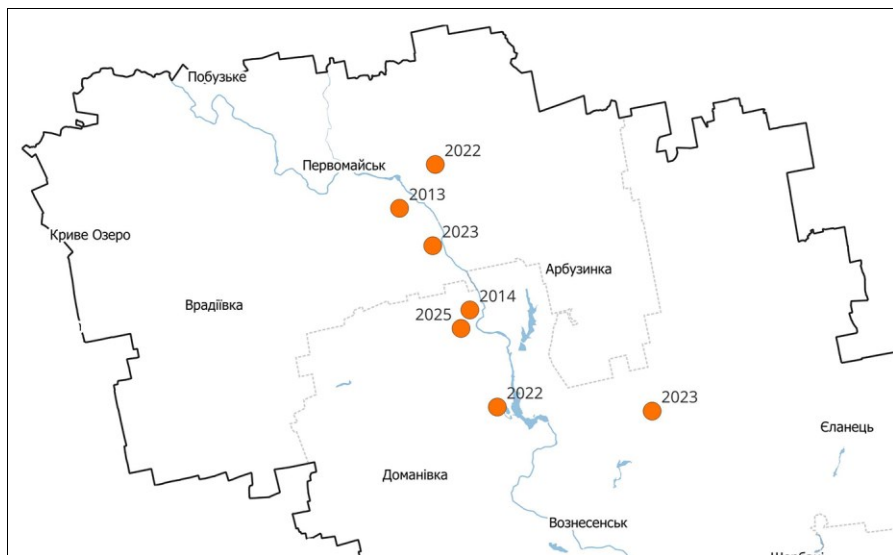
Рис. 1. Схема зустрічей Felis silvestris на Миколаївщині (пн.-зх. кут області).
